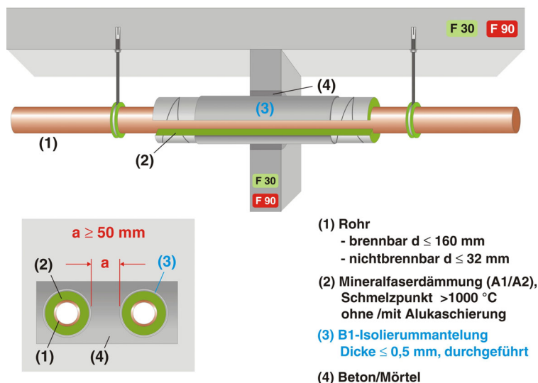
Bild 5: Anforderungen nach den Erleichterungen der Leitungsanlagen-Richtlinie Kapitel 4.2 bei Rohrdurchführungen mit nichtbrennbaren Mineralfaserdämmstoffen, Schmelzpunkt > 1000°C, inkl. einer B1-Isolierummantelung bis 0,5 mm Dicke
