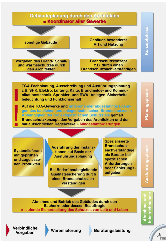
Bild 3 Entscheidungswege der brandschutztechnischen TGA-Planung
