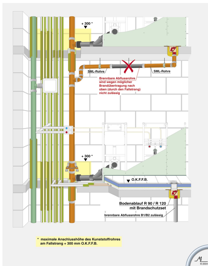
Bild 2 R90 klassifizierte Abschottung für SML-Rohre mit Anschlussmöglichkeit von brennbaren Rohren (siehe www.mlpartner.de <Download / Herstellerdokumente / Rockwool / überarbeitetes ABP für nichtbrennbare Rohre)
