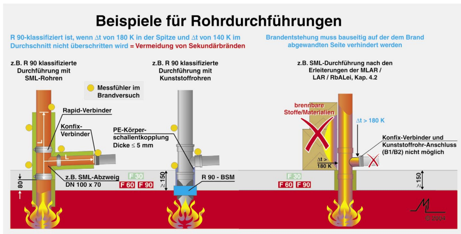
Bild 1 Vergleich von Abschottungsvarianten nach MLAR/LAR/RbALei
